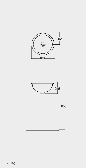
راك-إيما ٤٠ سم RAK-Emma Under Counter (W/O Overflow) 40 CM
