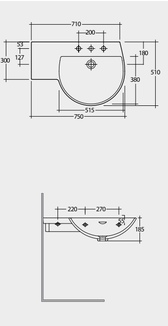
راك-ريزرفا وينغ يسار ٧٥ سم
