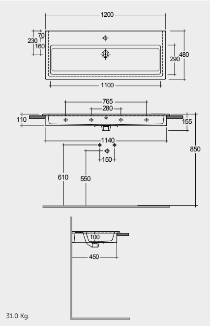
راك-مون ١٢٠ سم RAK-MOON 120 CM
