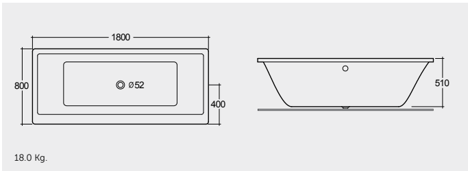
RAK-Metropolitan 180X80 CM راك-متروبوليتان ١٨٠X٨٠ سم
