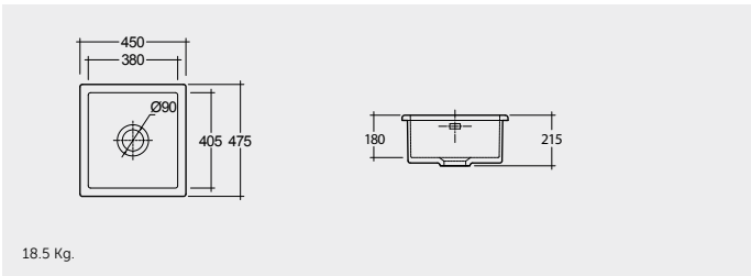
45 CM OC104AWHA External overflow optional نقبة تصريف الفائض اختياري
