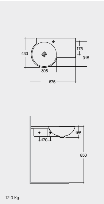
راك-جينا يمين ٦٧ سم
