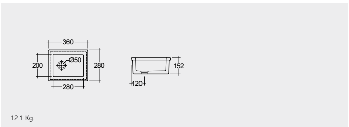
RAK-Lab Sink#3 58 CMراك-حوض مختبر#٣ ٥٨ سم
