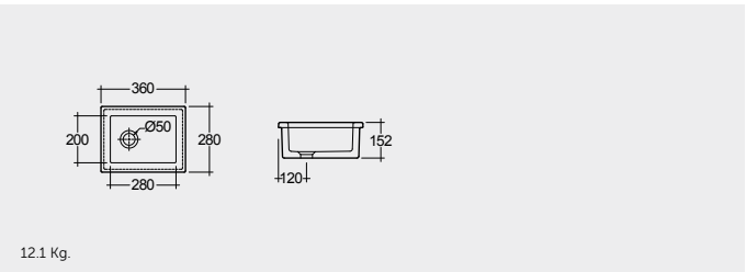
FIRE CLAY KITCHEN SINK 36 CM حوض مطبخ مصنوع من الطين الحراري ٣٦ سم
