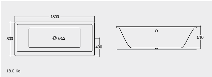
ACRYLIC DROP IN BATHTUB 180X80 CM حوض استحمام مدمج أكريليكي ١٨٠X٨٠ سم
