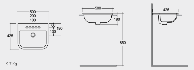
DROP IN WASH BASIN 50 CM حوض غسيل الوجه واليدين كاونتر سفلي ٥٠ سم
