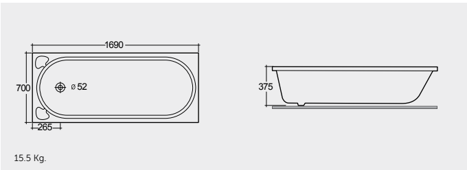
ACRYLIC DROP IN BATHTUB 169X70 CM حوض استحمام مدمج أكريليكي ١٦٩X٧٠ سم
