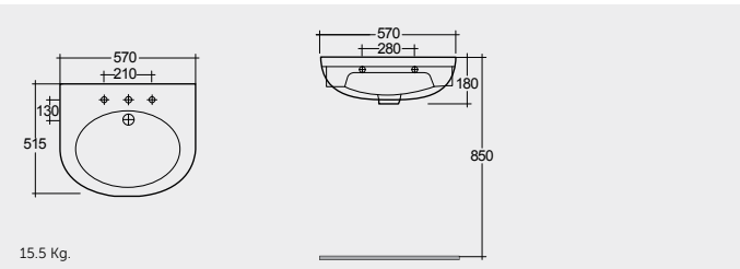
SEMI RECESSED WASH BASIN 57 CM حوض غسيل الوجه واليدين نصف مثبت علي الكاونتر ٥٧ سم
