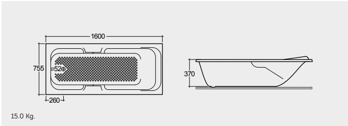
ACRYLIC DROP IN BATHTUB 160X75 CM حوض استحمام مدمج أكريليكي ١٦٠X٧٥ سم
