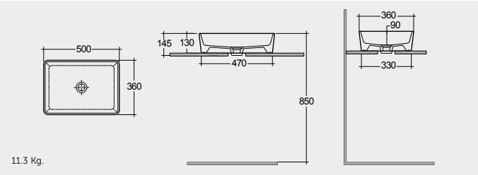
RECTANGULAR COUNTER TOP WASH BASIN 50 CM حوض غسيل الوجه واليدين كاونتر سطحي مستطيل ٥٠ سم
