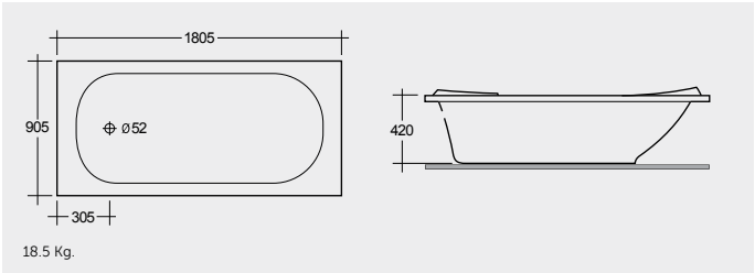
ACRYLIC DROP IN BATHTUB 180X90 CM حوض استحمام مدمج أكريليكي ١٨٠X٩٠ سم
