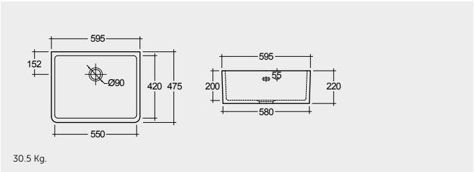
FIRE CLAY KITCHEN SINK 59 CM حوض مطبخ مصنوع من الطين الحراري ٥٩ سم
