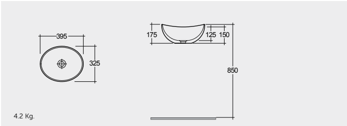
COUNTER TOP WASH BASIN BOWL 39 CM حوض غسيل الوجه واليدين كاونتر سطحي ٣٩ سم
