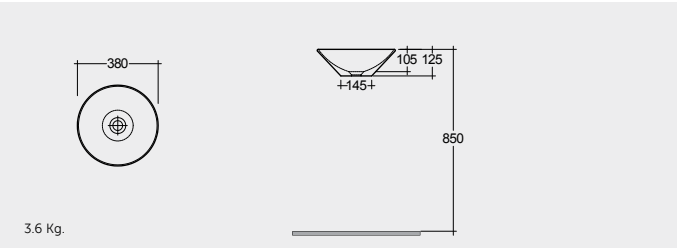
COUNTER TOP WASH BASIN 38 CM حوض غسيل الوجه واليدين كاونتر سطحي ٣٨ سم
