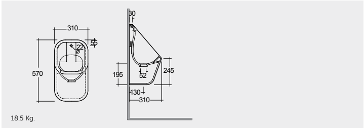
URINAL 31 CM مبولة ٣١ سم
