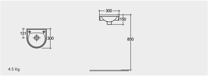
CLOAKROOM WASH BASIN 30 CM حوض غسيل الوجه واليدين لحمامات صغيرة ٣٠ سم
