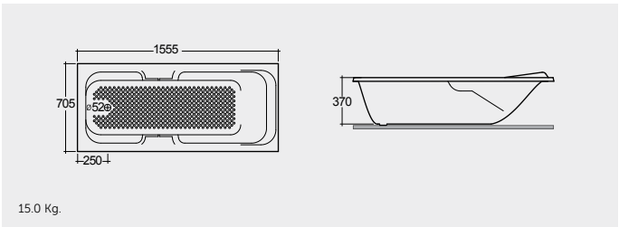
ACRYLIC DROP IN BATHTUB 155X70 CM حوض استحمام مدمج أكريليكي ١٥٥X٧٠ سم
