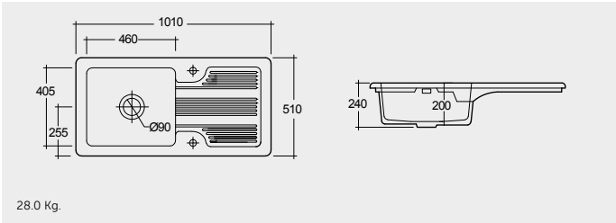
FIRE CLAY KITCHEN SINK 101 CM حوض مطبخ مصنوع من الطين الحراري ١٠١ سم
