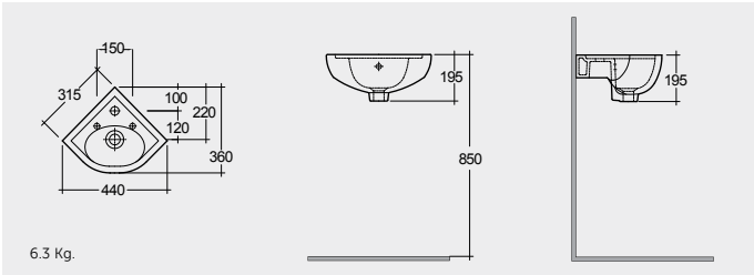
CORNER CLOAKROOM WASH BASIN 44 CM حوض غسيل الوجه واليدين زاوية لمراوض صغير ٤٤ سم
