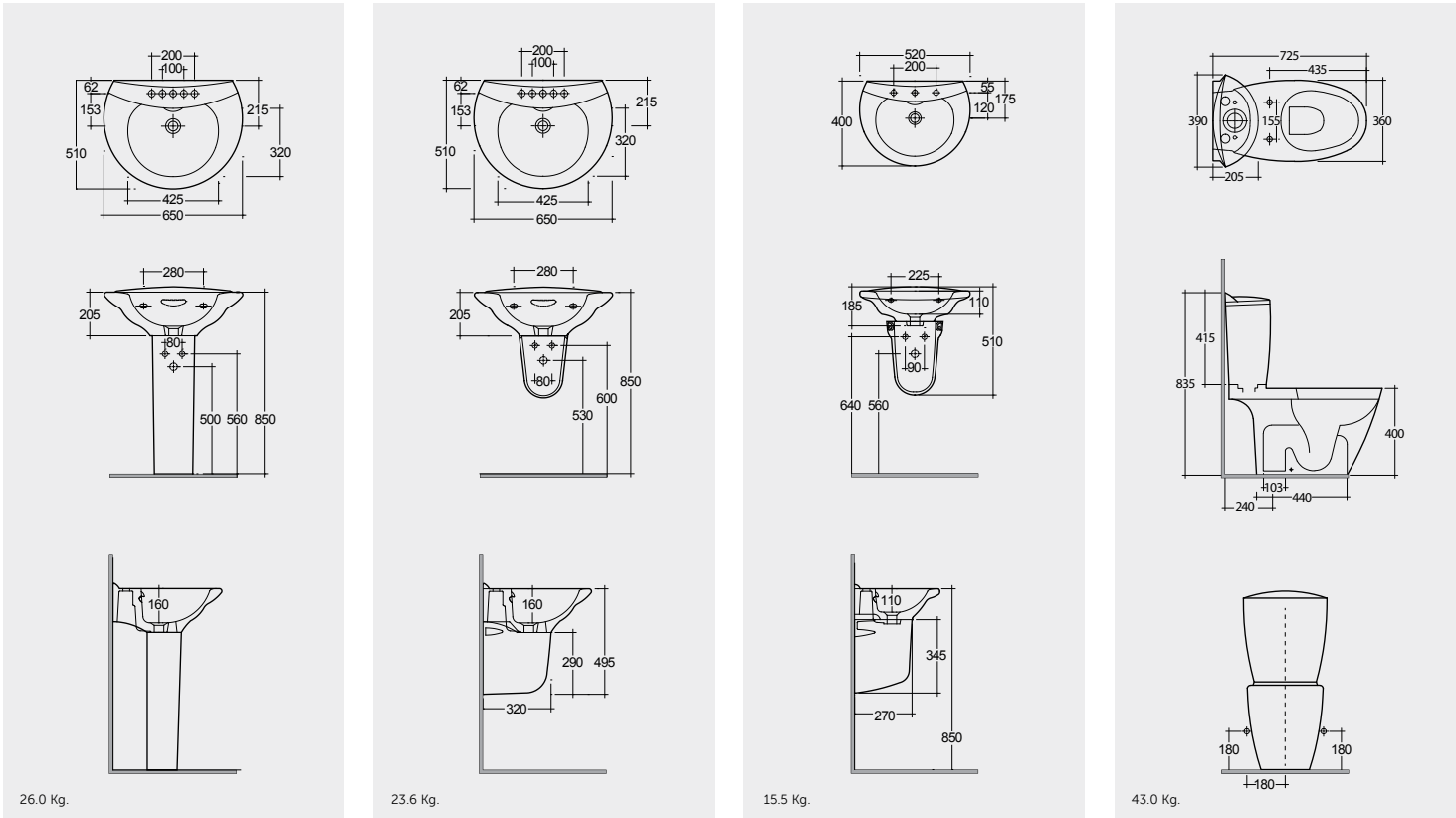
WASH BASIN WITH PEDESTAL 65 CM حوض غسيل الوجه واليدين بقاعدة ارتكاز كاملة ٦٥ سم WASH BASIN WITH HALF PEDESTAL 65 CM حوض غسيل الوجه واليدين بقاعدة نصف ارتكازية ٦٥ سم WASH BASIN WITH HALF PEDESTAL 52 CM حوض غسيل الوجه واليدين بقاعدة نصف ارتكازية ٥٢ سم CLOSE COUPLED WC (S) TRAP 72 CM حمامات متقارنة متقاربة بمحبس غلق مزدوج (إس) ٧٢ سم
