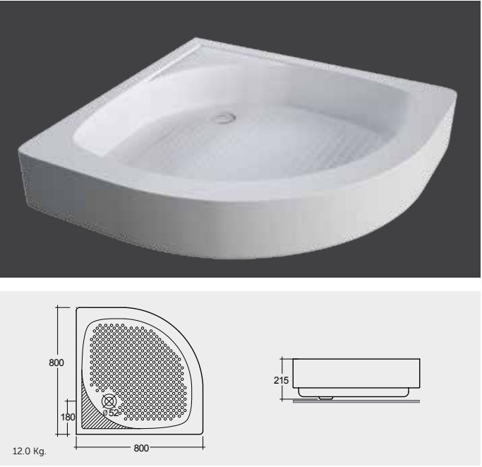
ACRYLIC SHOWER TRAY 80X80 CM حوض استحمام مسطح ٨٠X٨٠ سم
