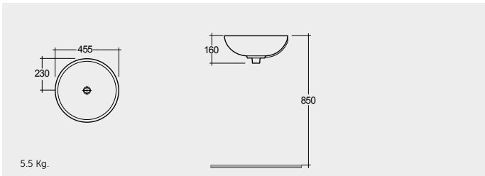
COUNTER TOP WASH BASIN BOWL 45 CM حوض غسيل الوجه واليدين كاونتر سطحي ٤٥ سم
