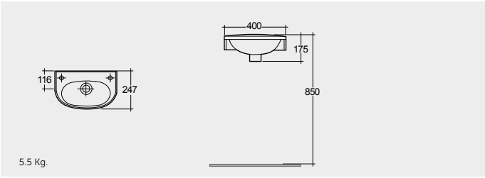
CLOAKROOM WASH BASIN 44 CM حوض غسيل الوجه واليدين لحمامات صغيرة ٤٤ سم
