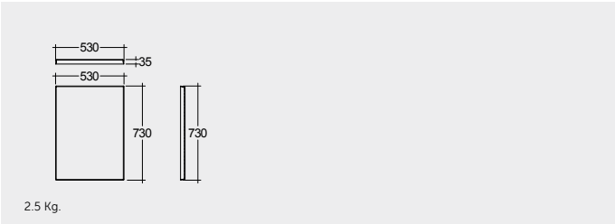
ACRYLIC BATHTUB SHORT SIDE PANEL 170 CM ألواح جانبية قصيرة لحوض استحمام مدمج أكريليكي ١٧٠ سم
