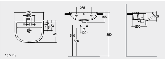
SEMI RECESSED WASH BASIN 55 CM حوض غسيل الوجه واليدين نصف مثبت علي الكاونتر ٥٥ سم
