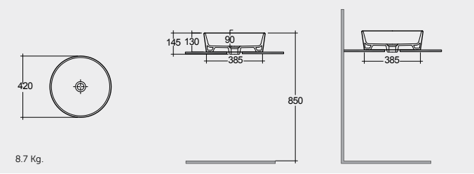
ROUND COUNTER TOP WASH BASIN 42 CM حوض غسيل الوجه واليدين كاونتر سطحي دائري ٤٢ سم
