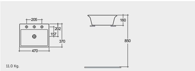
COUNTER TOP WASH BASIN 47 CM حوض غسيل الوجه واليدين كاونتر سطحي ٤٧ سم
