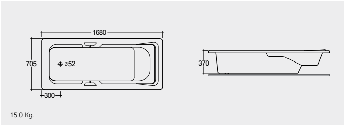
ACRYLIC DROP IN BATHTUB 170X70 CM حوض استحمام مدمج أكريليكي ١٧٠X٧٠ سم
