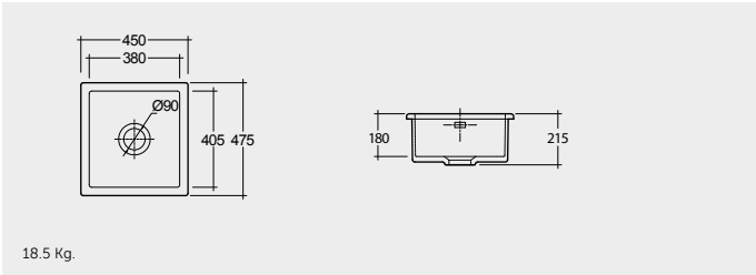
FIRE CLAY KITCHEN SINK 45 CM حوض مطبخ مصنوع من الطين الحراري ٤٥ سم
