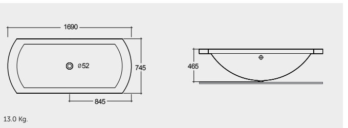
ACRYLIC DROP IN BATHTUB 169X74.5 CM حوض استحمام مدمج أكريليكي ١٦٩X٧٤.٥ سم
