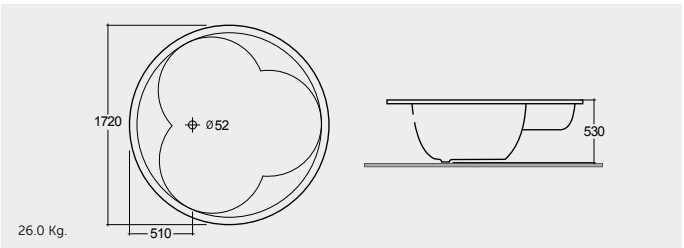
ACRYLIC DROP IN BATHTUB 172X172 CM حوض استحمام مدمج أكريليكي ١٧٢X١٧٢ سم
