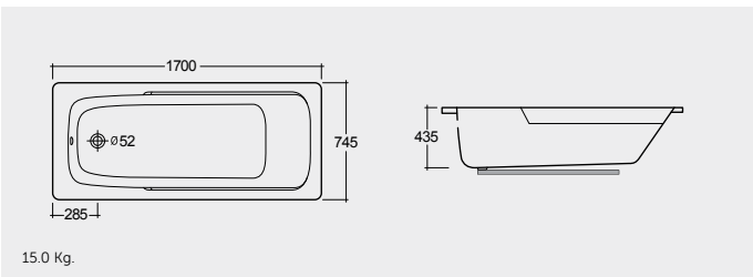
ACRYLIC DROP IN BATHTUB 170X74 CM حوض استحمام مدمج أكريليكي ١٧٠X٧٤ سم
