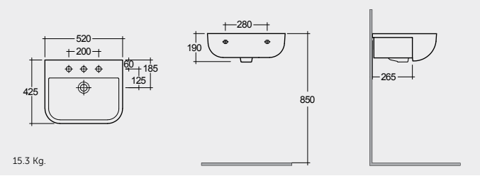
SEMI RECESSED WASH BASIN 52 CM حوض غسيل الوجه واليدين نصف مثبت علي الكاونتر ٥٢ سم
