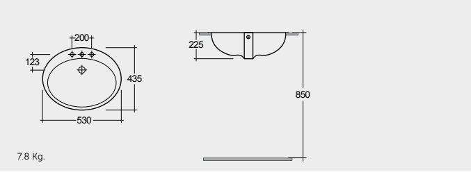
DROP IN WASH BASIN 53 CM حوض غسيل الوجه واليدين كاونتر سفلي ٥٣ سم
