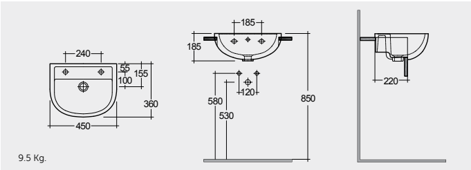
SEMI RECESSED WASH BASIN 45 CM حوض غسيل الوجه واليدين نصف مثبت علي الكاونتر ٤٥ سم
