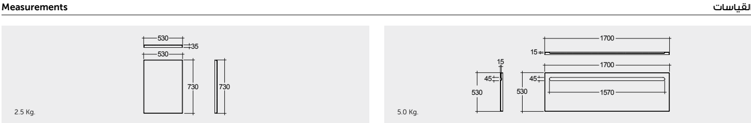
ACRYLIC BATHTUB SHORT SIDE PANEL 170 CM ألواح جانبية قصيرة لحوض استحمام أكريليكي ١٧٠ سم ACRYLIC BATHTUB LONG SIDE PANEL 170 CM ألواح جانبية طويلة لحوض استحمام أكريليكي ١٧٠ سم
