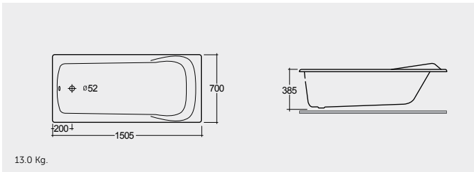
ACRYLIC DROP IN BATHTUB 150X70 CM حوض استحمام مدمج أكريليكي ١٥٠X٧٠ سم
