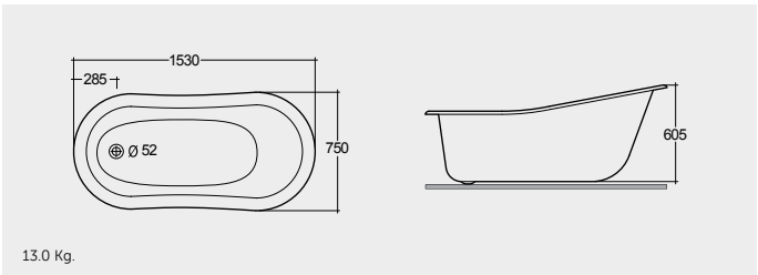
ACRYLIC DROP IN BATHTUB 153X75 CM حوض استحمام مدمج أكريليكي ١٥٣X٧٥ سم
