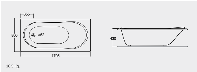
ACRYLIC DROP IN BATHTUB 170X80 CM حوض استحمام مدمج أكريليكي ١٧٠X٨٠ سم
