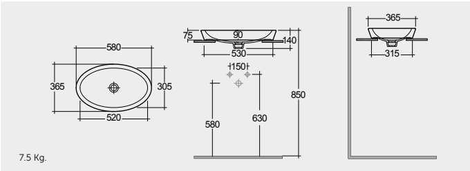
COUNTER TOP WASH BASIN 58 CM حوض غسيل الوجه واليدين كاونتر سطحي ٥٨ سم
