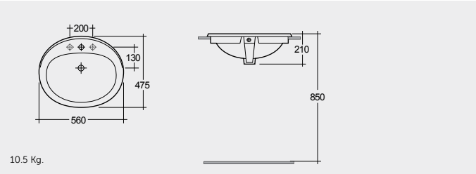
DROP IN WASH BASIN 56 CM حوض غسيل الوجه واليدين كاونتر سفلي ٥٦ سم
