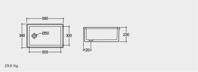
FIRE CLAY KITCHEN SINK 58 CM حوض مطبخ مصنوع من الطين الحراري ٥٨ سم
