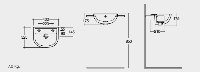
SEMI RECESSED WASH BASIN 40 CM حوض غسيل الوجه واليدين نصف مثبت علي الكاونتر ٤٠ سم
