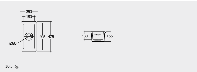
FIRE CLAY KITCHEN SINK 25 CM حوض مطبخ مصنوع من الطين الحراري ٢٥ سم
