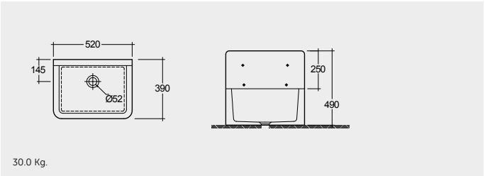
CLEANER SINK 52 CM حوض تنظيف ٥٢ سم
