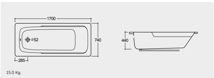
ACRYLIC DROP IN BATHTUB DELUXE 170X74 CM حوض استحمام مدمج أكريليكي فاخر ١٧٠X٧٤ سم
