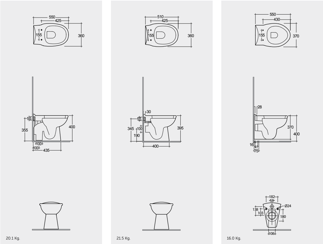
ABS Karla seat & cover Soft close also available Karla urea seat and cover مقعد وغطاء إيه بي إس كارلا متوفر بخيار سوفت كلوز مقعد وغطاء كارلا يوريا ABS Karla seat & cover Soft close also available Karla urea seat and cover مقعد وغطاء إيه بي إس كارلا متوفر بخيار سوفت كلوز مقعد وغطاء كارلا يوريا ABS Karla seat & cover Soft close also available Karla urea seat and cover مقعد وغطاء إيه بي إس كارلا متوفر بخيار سوفت كلوز مقعد وغطاء كارلا يوريا
