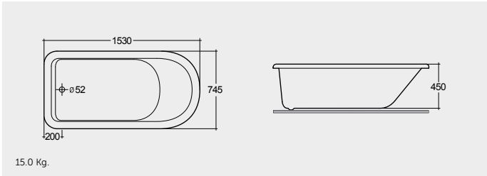
ACRYLIC DROP IN BATHTUB 153X74 CM حوض استحمام مدمج أكريليكي ١٥٣X٧٤ سم
