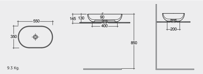
OVAL COUNTER TOP WASH BASIN 55 CM حوض غسيل الوجه واليدين كاونتر سطحي بيضوي ٥٥ سم
