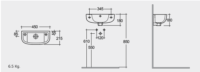
CLOAKROOM WASH BASIN 45 CM حوض غسيل الوجه واليدين لحمامات صغيرة ٤٥ سم
