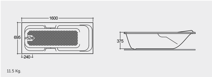
ACRYLIC DROP IN BATHTUB 160X70 CM حوض استحمام مدمج أكريليكي ١٦٠X٧٠ سم
