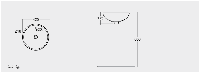
COUNTER TOP WASH BASIN BOWL W/OF 42 CM حوض غسيل الوجه واليدين كاونتر سطحي ٤٢ سم
