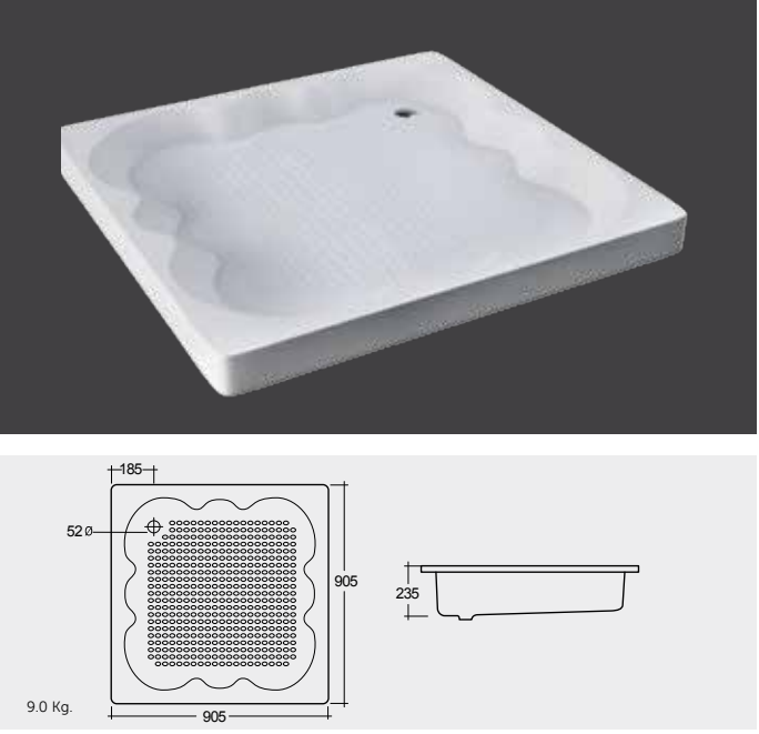
ACRYLIC SHOWER TRAY 90X90 CM حوض استحمام مسطح ٩٠X٩٠ سم
