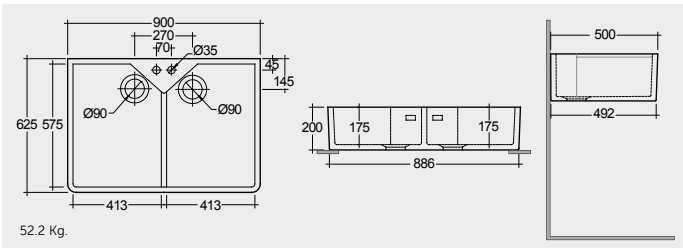
FIRE CLAY KITCHEN SINK 90 CM حوض مطبخ مصنوع من الطين الحراري ٩٠ سم
