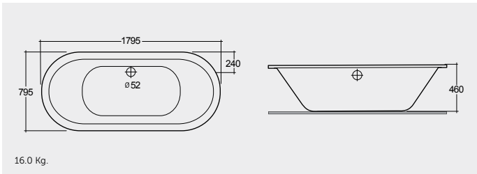
ACRYLIC DROP IN BATHTUB 179X79 CM حوض استحمام مدمج أكريليكي ١٧٩X٧٩ سم
