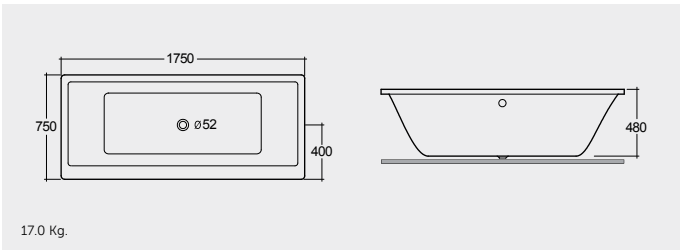
ACRYLIC DROP IN BATHTUB 175X75 CM حوض استحمام مدمج أكريليكي ١٧٥X٧٥ سم
