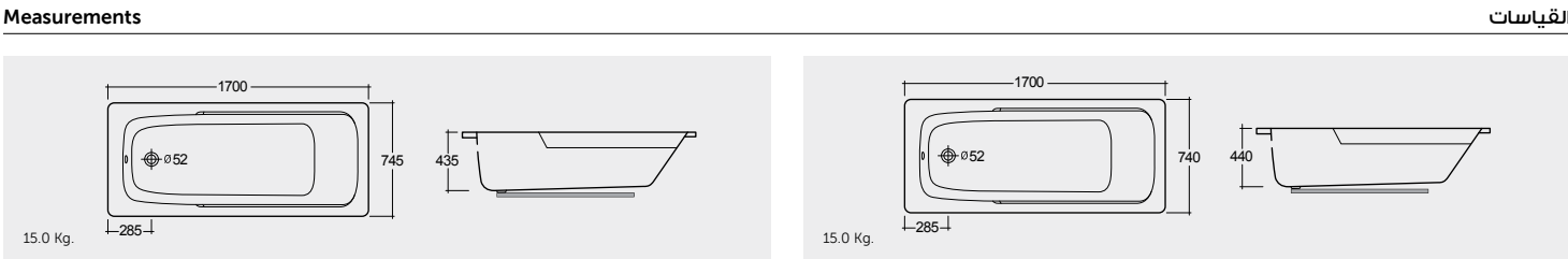
ACRYLIC DROP IN BATHTUB 170X74 CM حوض استحمام مدمج أكريليكي ١٧٠.X٧٤ سم DELUXE ACRYLIC DROP IN BATHTUB 170X74 CM حوض استحمام مدمج أكريليكي فاخر ١٧٠.X٧٤ سم
