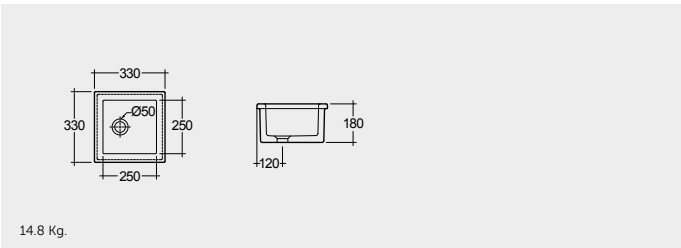
FIRE CLAY KITCHEN SINK 33 CM حوض مطبخ مصنوع من الطين الحراري ٣٣ سم
