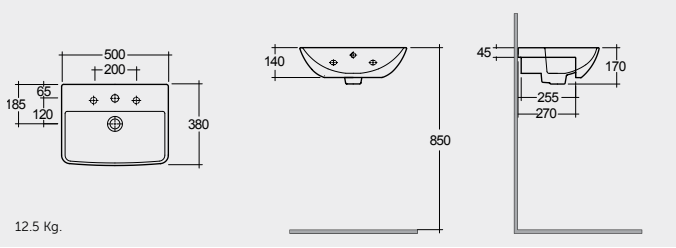
SEMI RECESSED WASH BASIN 50 CM حوض غسيل الوجه واليدين نصف مثبت علي الكاونتر ٥٠ سم
