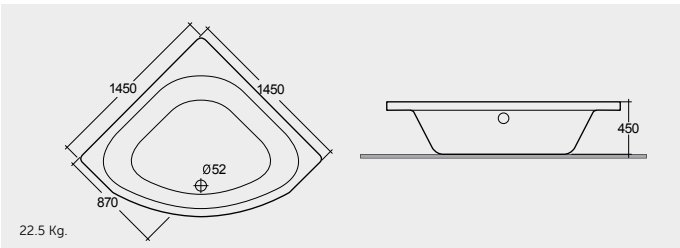
ACRYLIC DROP IN BATHTUB 145X145 CM حوض استحمام مدمج أكريليكي ١٤٥X١٤٥ سم
