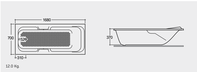
ACRYLIC DROP IN BATHTUB 168X70 CM حوض استحمام مدمج أكريليكي ١٦٨X٧٠ سم
