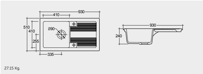
FIRE CLAY KITCHEN SINK 93 CM حوض مطبخ مصنوع من الطين الحراري ٩٣ سم
