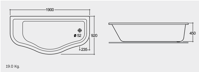
ACRYLIC DROP IN BATHTUB 190X92 CM حوض استحمام مدمج أكريليكي ١٩٠X٩٢ سم
