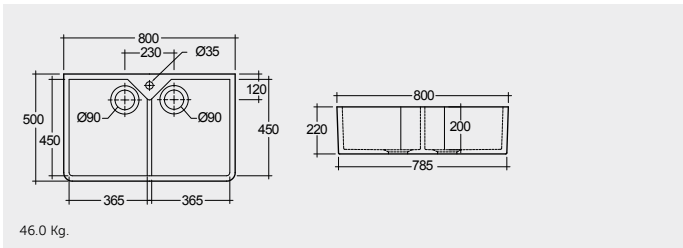
FIRE CLAY KITCHEN SINK 80 CM حوض مطبخ مصنوع من الطين الحراري ٨٠ سم
