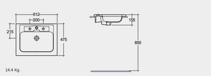
DROP IN WASH BASIN 61 CM حوض غسيل الوجه واليدين كاونتر سفلي ٦١ سم
