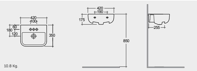
SEMI RECESSED WASH BASIN 42 CM حوض غسيل الوجه واليدين نصف مثبت علي الكاونتر ٤٢ سم
