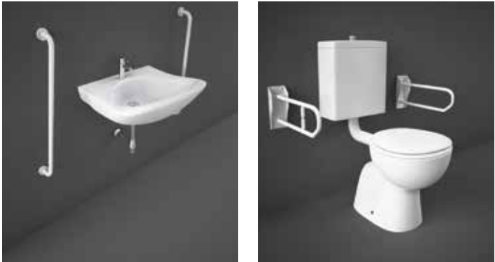
BELLA DISABLED WALL HUNG WASH BASIN 61 CM بيلا ديس إيبولد حوض غسيل الوجه واليدين للتعليق على الحائط ٦١ سم BELLA DISABLED CLOSE COUPLED LINK SUITE WC (S) TRAP 61 CM بيلا ديس إيبولد حمامات متقاربة متقاربة بمحبس غلق مزدوج (اس) ٦١ سم
