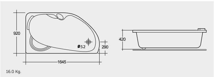
ACRYLIC DROP IN BATHTUB 164X92 CM حوض استحمام مدمج أكريليكي ١٦٤X٩٢ سم
