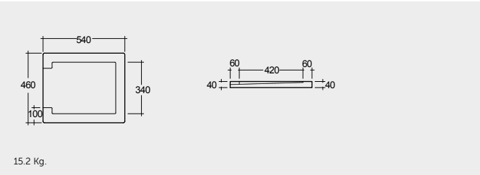
DRAIN BOARD 54 CM لوح تجفيف ٥٤ سم
