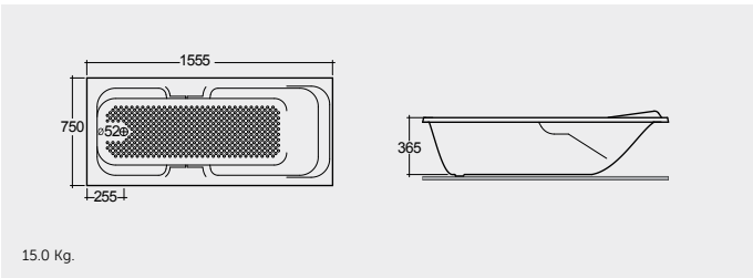
ACRYLIC DROP IN BATHTUB 155X75 CM حوض استحمام مدمج أكريليكي ١٥٥X٧٥ سم
