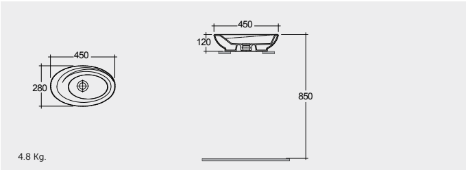
COUNTER TOP WASH BASIN 45 CM حوض غسيل الوجه واليدين كاونتر سطحي ٤٥ سم
