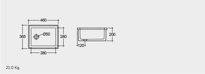
FIRE CLAY KITCHEN SINK 46 CM حوض مطبخ مصنوع من الطين الحراري ٤٦ سم
