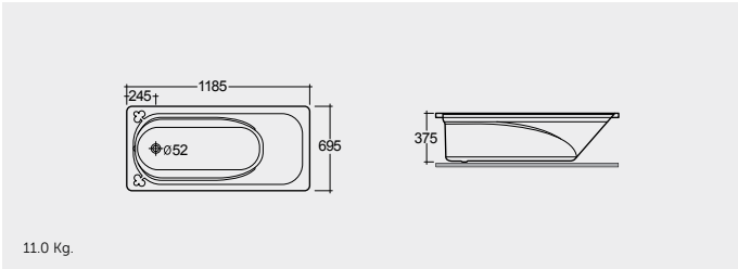
ACRYLIC DROP IN BATHTUB 118X69 CM حوض استحمام مدمج أكريليكي ١١٨X٦٩ سم
