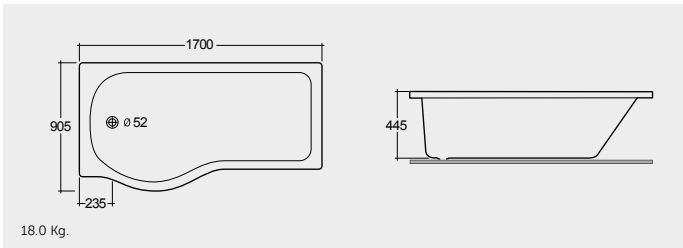
ACRYLIC DROP IN BATHTUB 170X90 CM حوض استحمام مدمج أكريليكي ١٧٠X٩٠ سم
