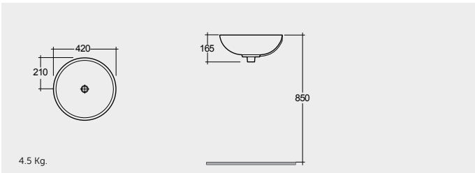
COUNTER TOP WASH BASIN BOWL 42 CM حوض غسيل الوجه واليدين كاونتر سطحي ٤٢ سم
