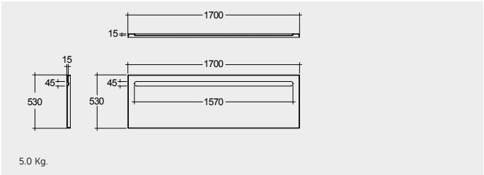
ACRYLIC BATHTUB LONG SIDE PANEL 170 CM ألواح جانبية طويلة لحوض استحمام مدمج أكريليكي ١٧٠ سم
