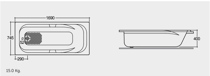
ACRYLIC DROP IN BATHTUB 169X74 CM حوض استحمام مدمج أكريليكي ١٦٩X٧٤ سم
