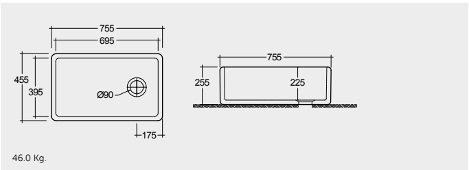
FIRE CLAY KITCHEN SINK 75 CM حوض مطبخ مصنوع من الطين الحراري ٧٥ سم
