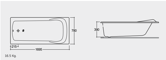
ACRYLIC DROP IN BATHTUB 169X78 CM حوض استحمام مدمج أكريليكي ١٦٩X٧٨ سم
