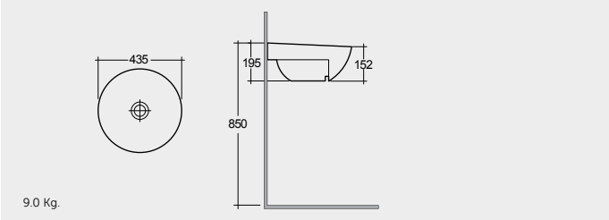
SEMI RECESSED WASH BASIN 43 CM حوض غسيل الوجه واليدين نصف مثبت علي الكاونتر ٤٣ سم
