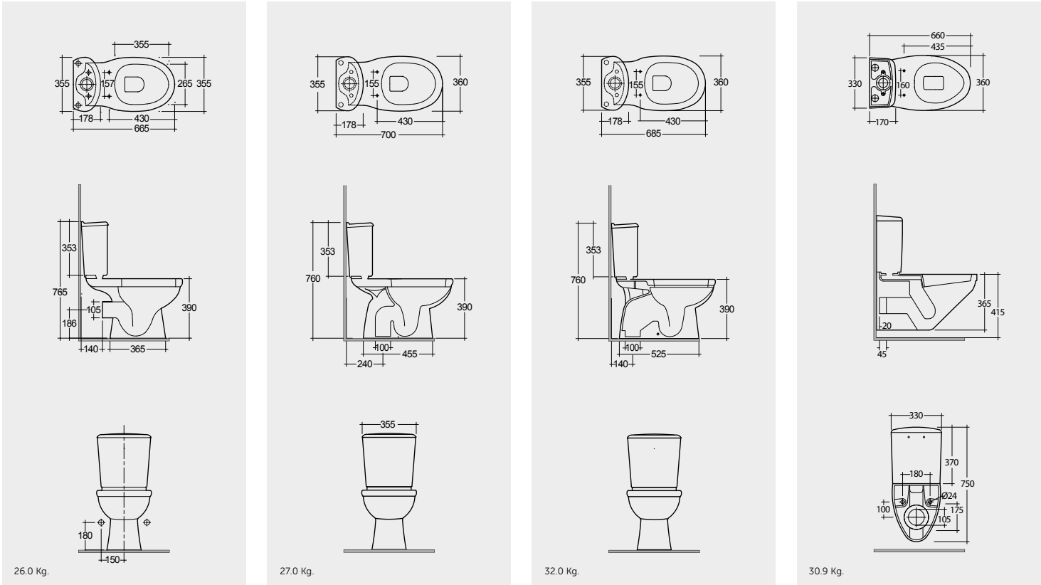
ABS Karla seat & cover Soft close also available Karla urea seat and cover مقعد وغطاء إيه بي إس كارلا متوفر بخيار سوفت كلوز مقعد وغطاء كارلا يوريا ABS Karla seat & cover Soft close also available Karla urea seat and cover مقعد وغطاء إيه بي إس كارلا متوفر بخيار سوفت كلوز مقعد وغطاء كارلا يوريا ABS Karla seat & cover Soft close also available Karla urea seat and cover مقعد وغطاء إيه بي إس كارلا متوفر بخيار سوفت كلوز مقعد وغطاء كارلا يوريا ABS Karla seat & cover Soft close also available Karla urea seat and cover مقعد وغطاء إيه بي إس كارلا متوفر بخيار سوفت كلوز مقعد وغطاء كارلا يوريا
